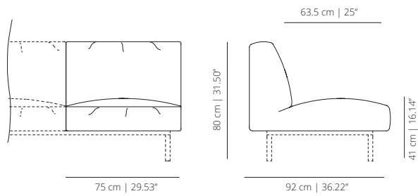
SISMPS module avec dossier medium
