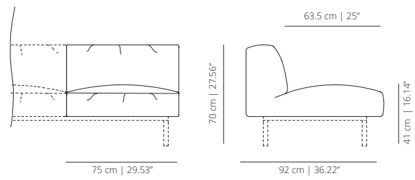
SISBPS module avec dossier bas
