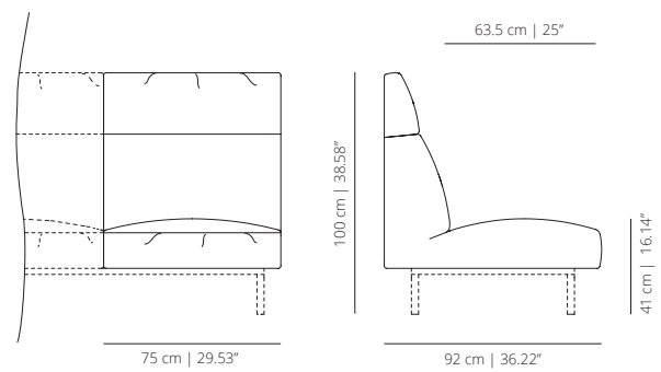
SISAPS module avec dossier haute
